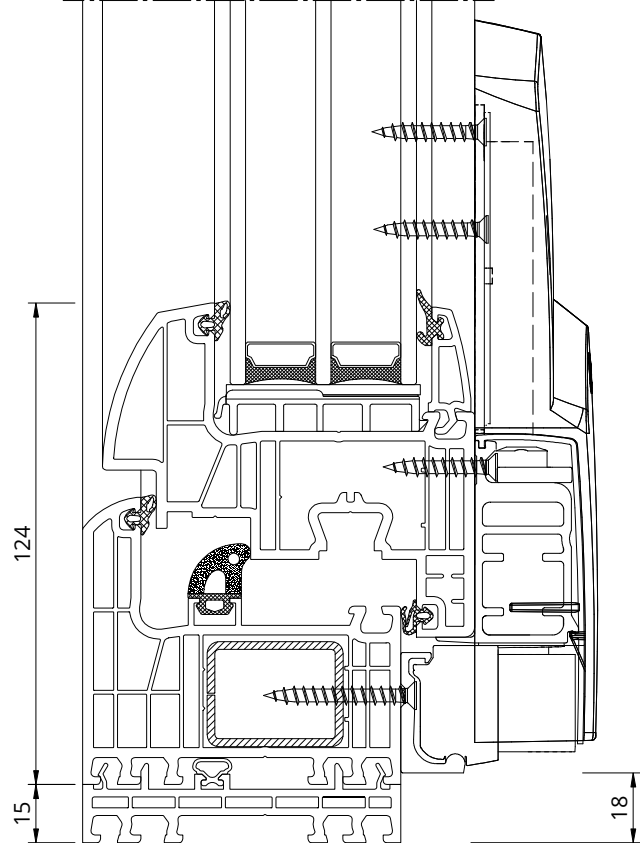
B - B
