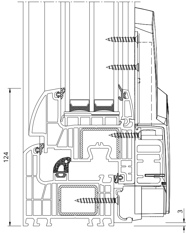
B - B
